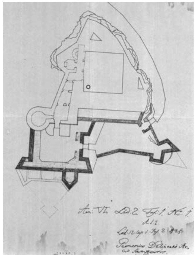
- Pôdorys prestavby Pajštúna. Výkres z prvej polovice 17. storočia. Vyčiernená časť je novostavba. -
